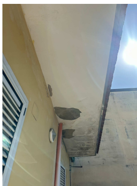
Solaio di copertura
